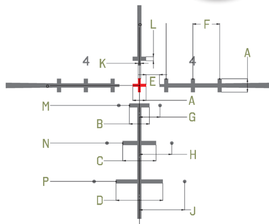
Dimensione de la cubierta en MOA para aumento mín./máx.
